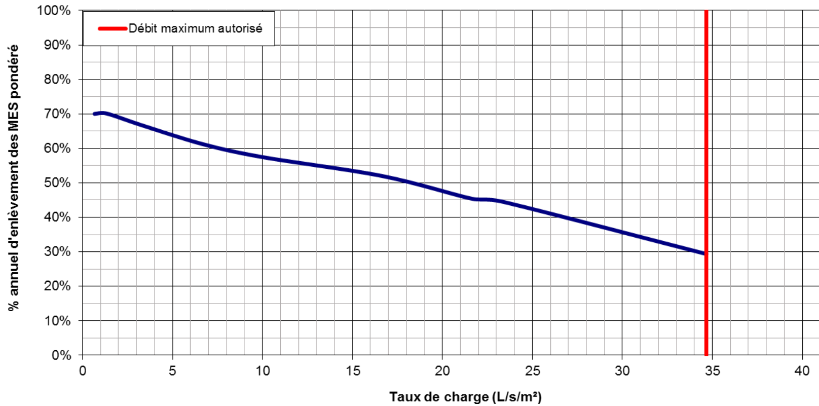
Figure 1 Performance annuelle d'enlèvement des matières en suspension (MES) pour différents débits. La performance tient compte des facteurs de pondération (voir l'article 6 de la fiche d'information Éléments considérés lors de l'évaluation de performance des technologies commerciales de type « séparateurs hydrodynamiques » effectuée par le Ministère ).
