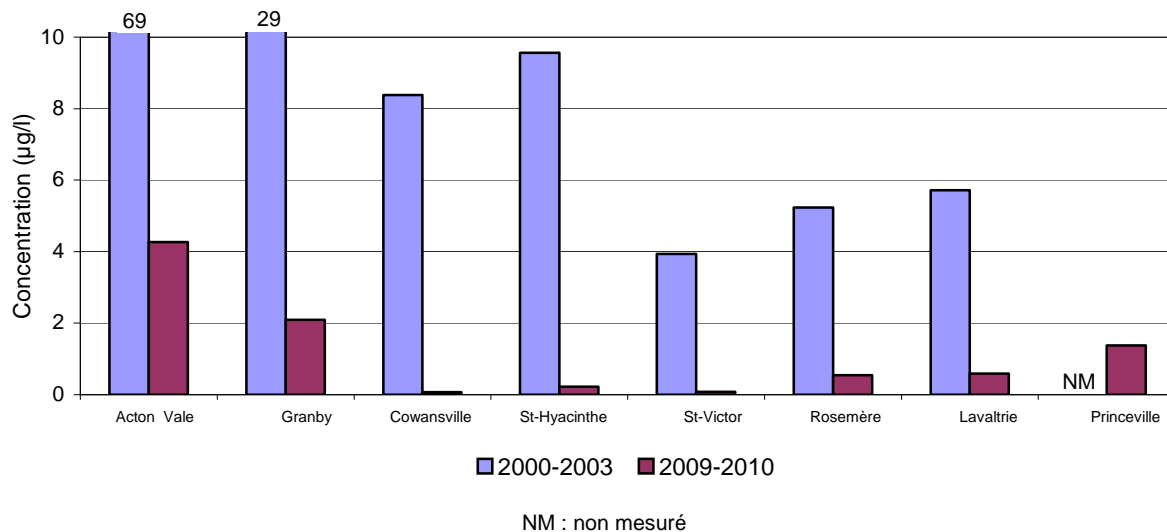
Figure 5 Concentrations médianes de nonylphénols éthoxylés et carboxylés totaux (NP1-17EO + NP1-2EC) aux huit stations d'échantillonnage
